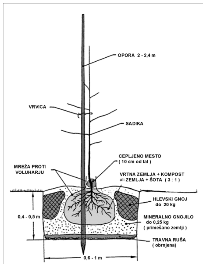
Skica sajenja sadnega drevja
